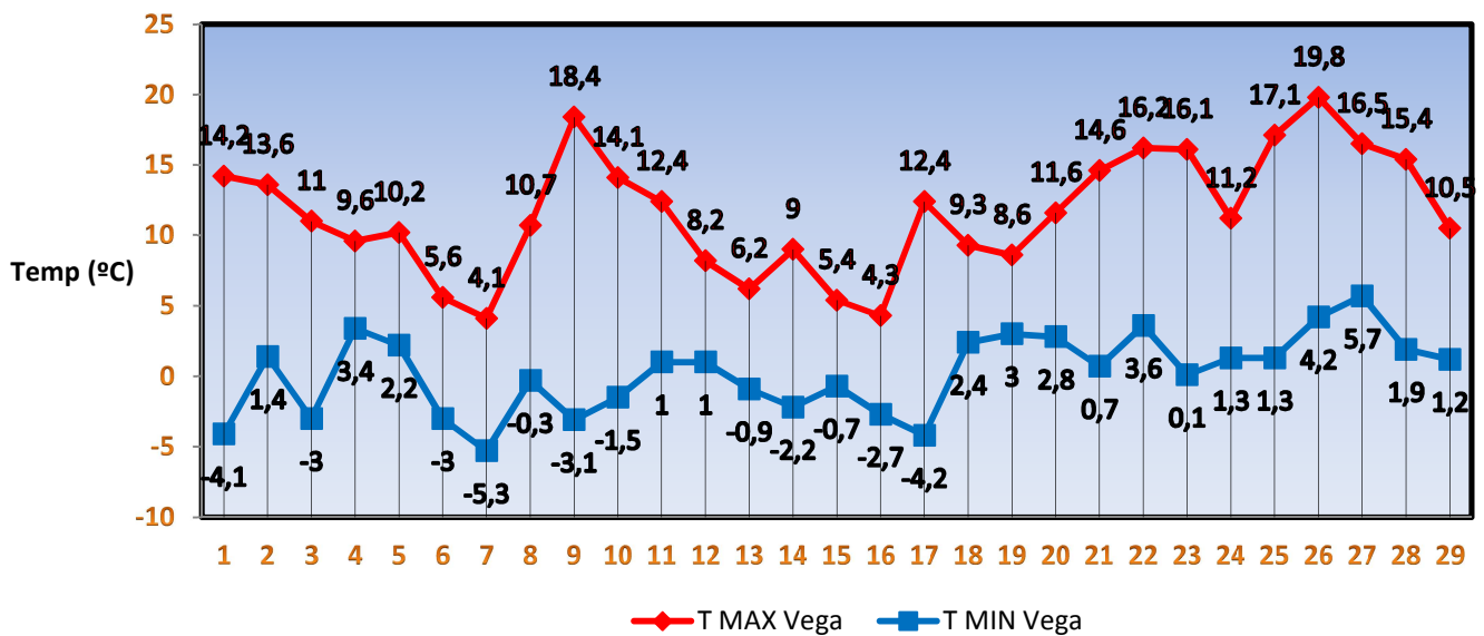
Gráfico 1. Evolución temperaturas Máx. y Mín. Abril 2012. (Fuente www.meteoalcaladelaselva.com )
