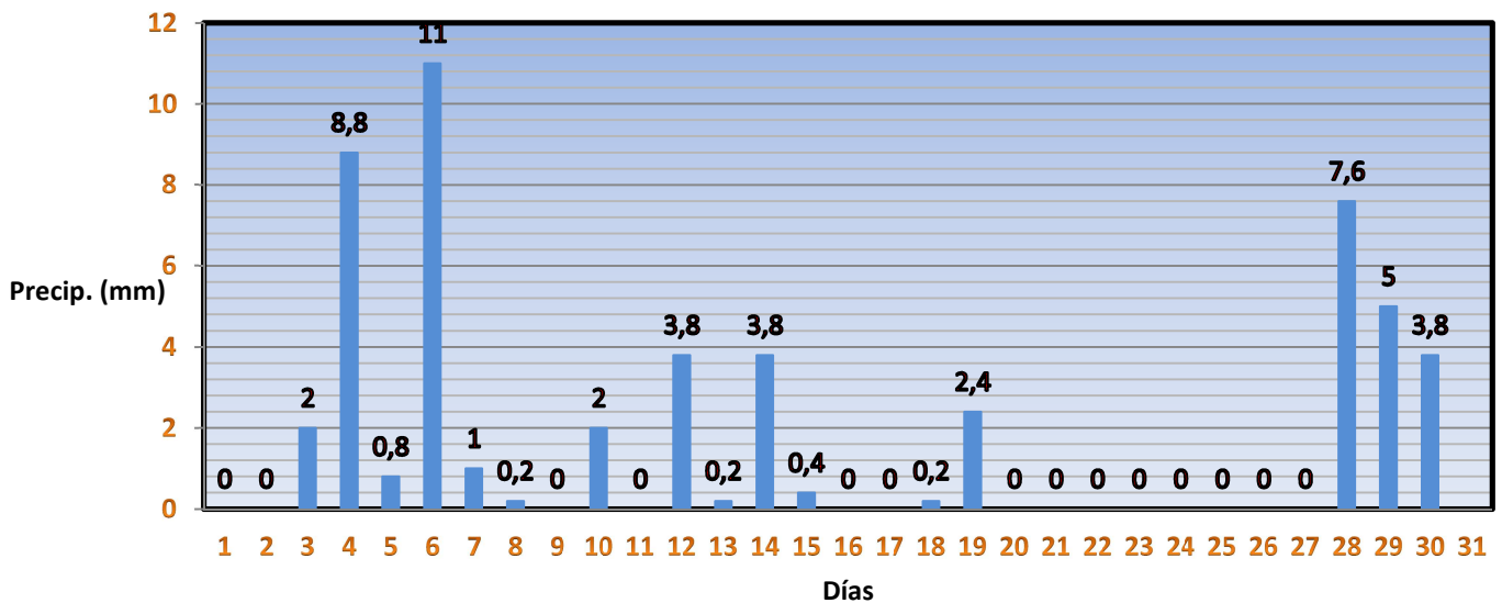
Gráfico 2. Precipitaciones diarias registradas. Totales acumulados. Abril 2012.
